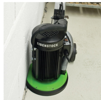
Mulighed for kantenær slibning
